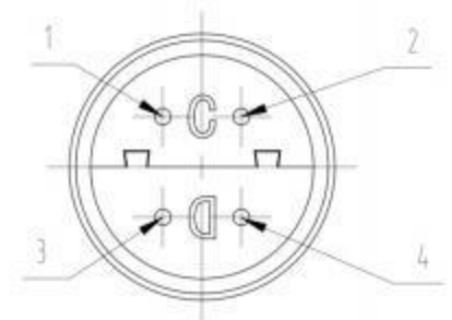
图5：接线定义示意图
